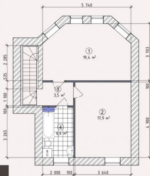
План 2-го этажа
