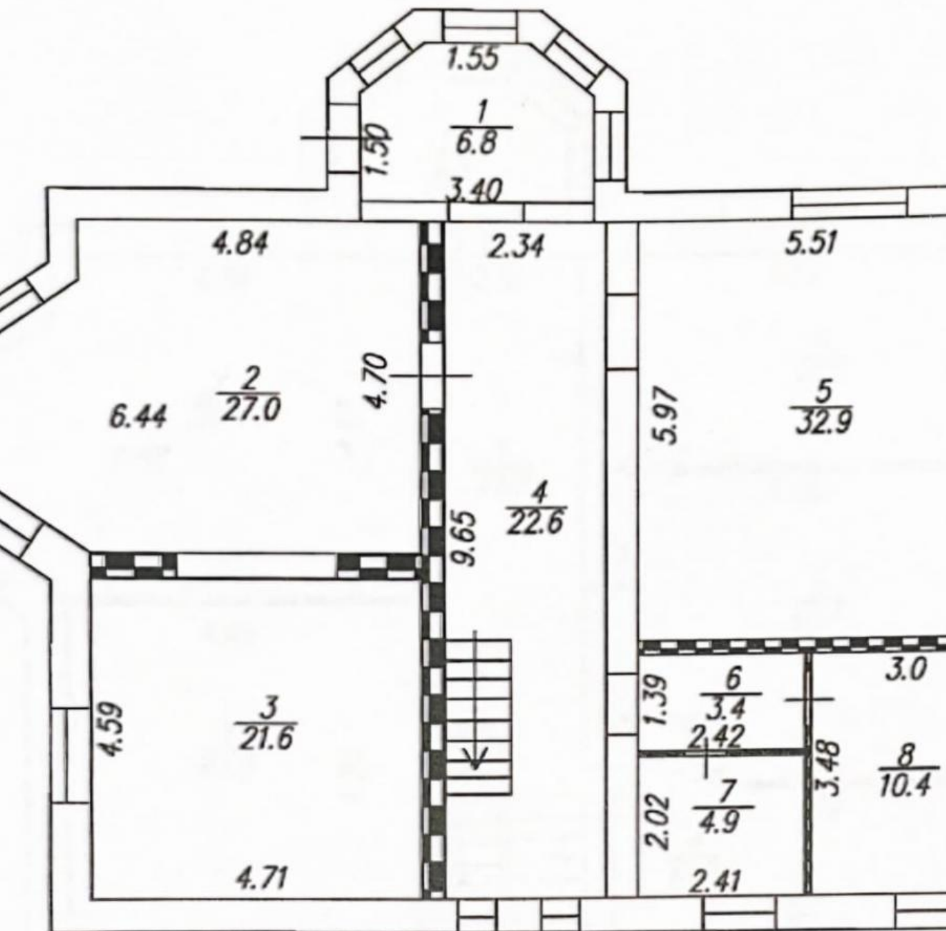
1-й этаж
